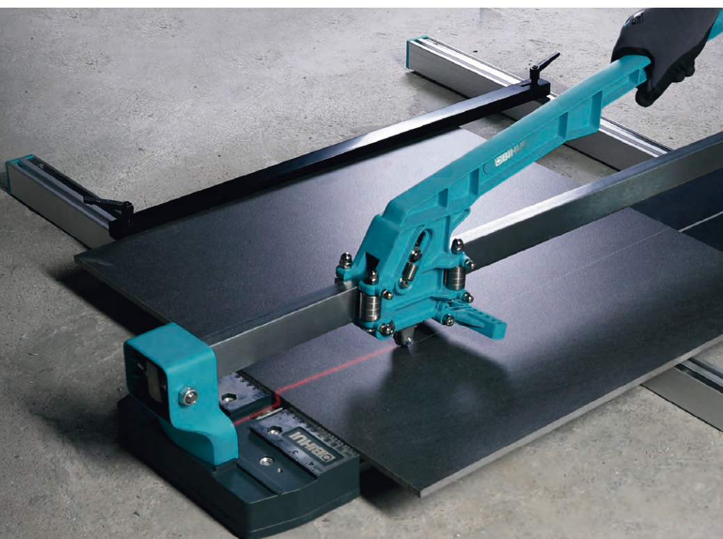
Cornice di taglio regolabile Adjustable cutting frame Long lifetime scoring wheel
